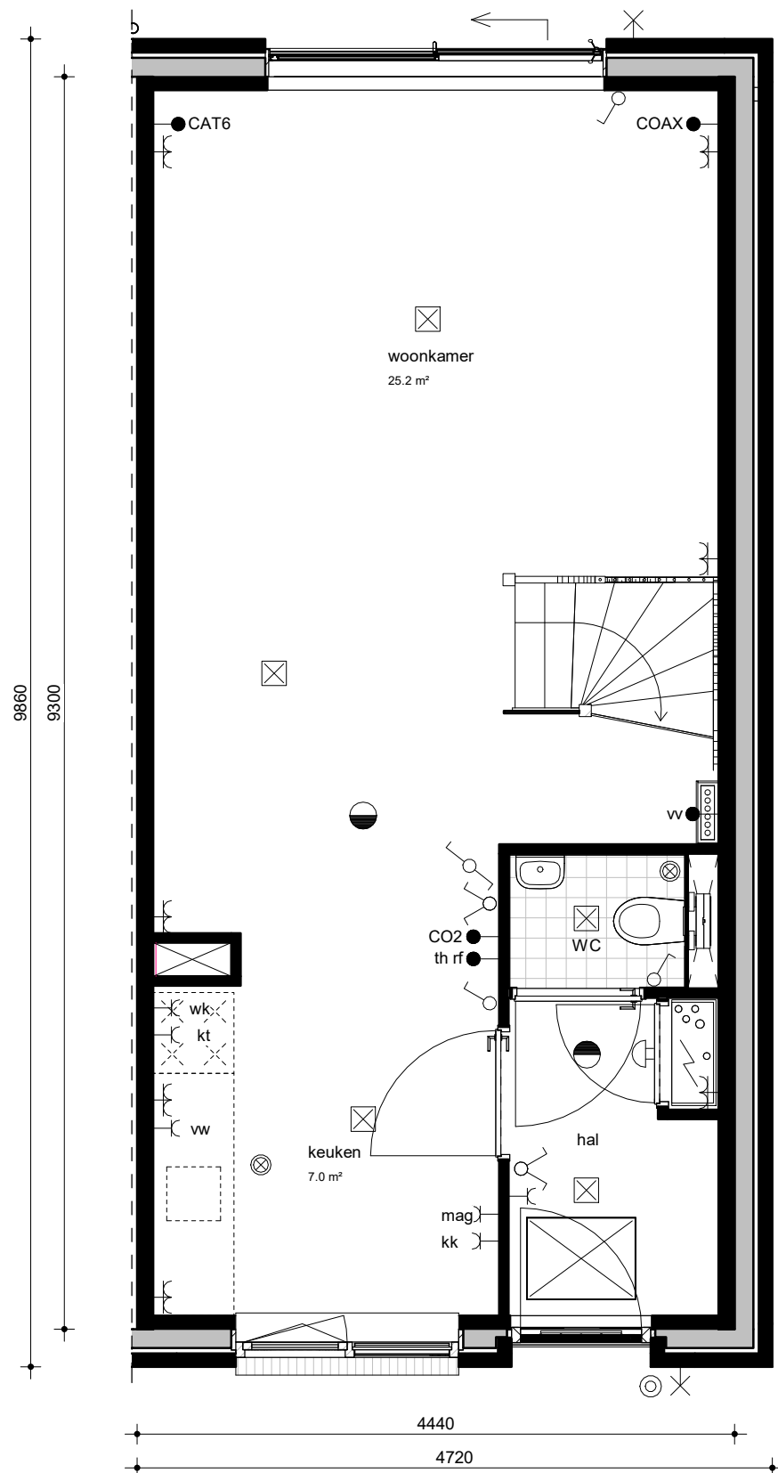
begane grond 1 : 50
